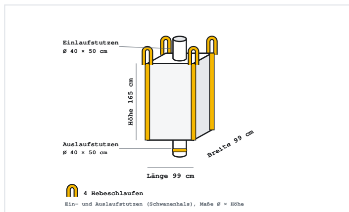
Maßzeichnung mit Abmessungen (Außenmaße, schematisch)
